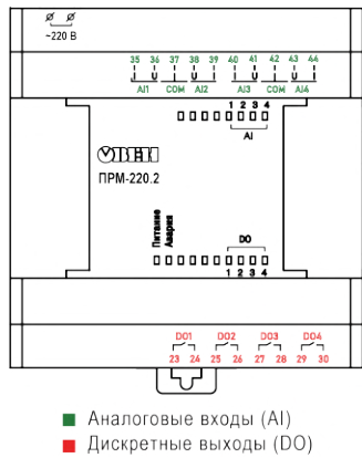
Рисунок 7.9 – Расположение и цветовая маркировка клемм ПРМ–2
