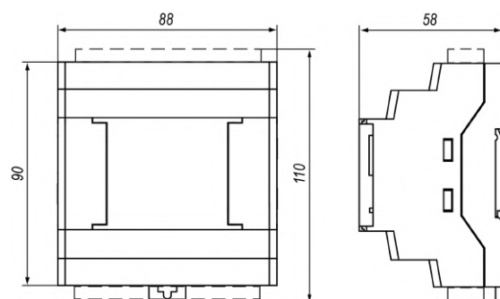
Рисунок 7.5 – Габаритные размеры
