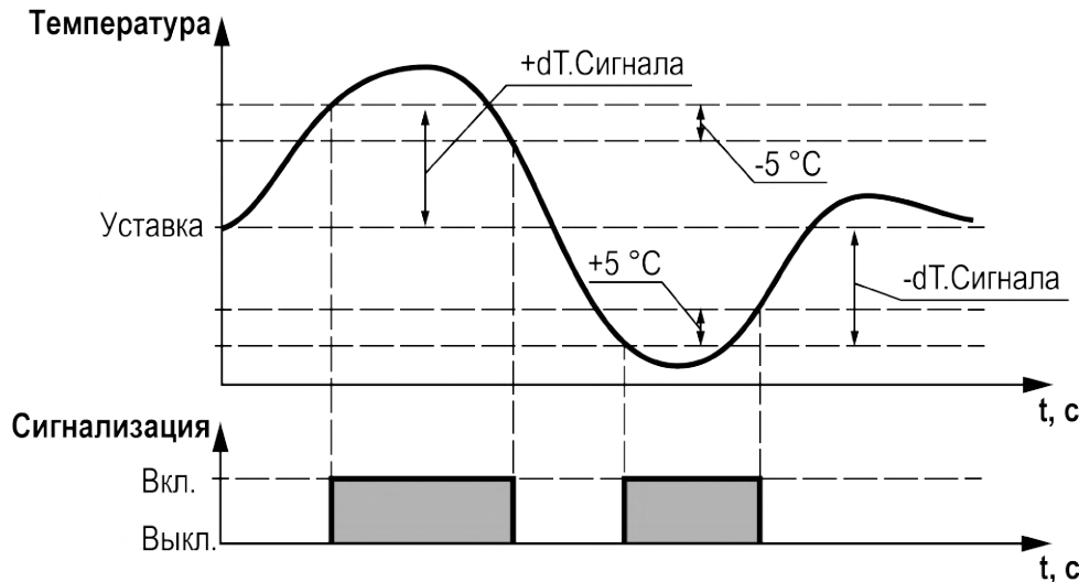
Рисунок 10.1 – Работа сигнализации по температуре
