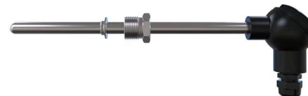
Рисунок Б.3 – ДТСxx5 с подвижным штуцером (модели 035, 045, 145 и 335)
