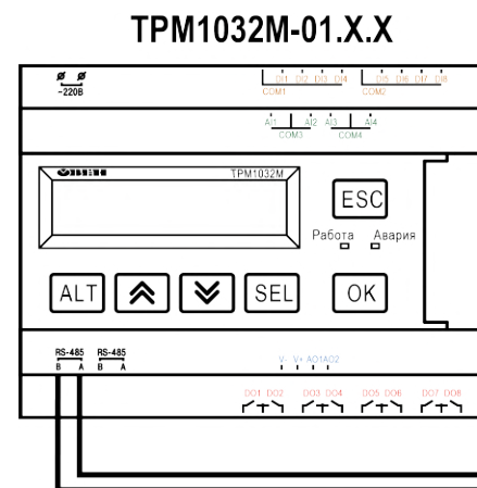
Рисунок 7.20 – Схема подключения для диспетчеризации
